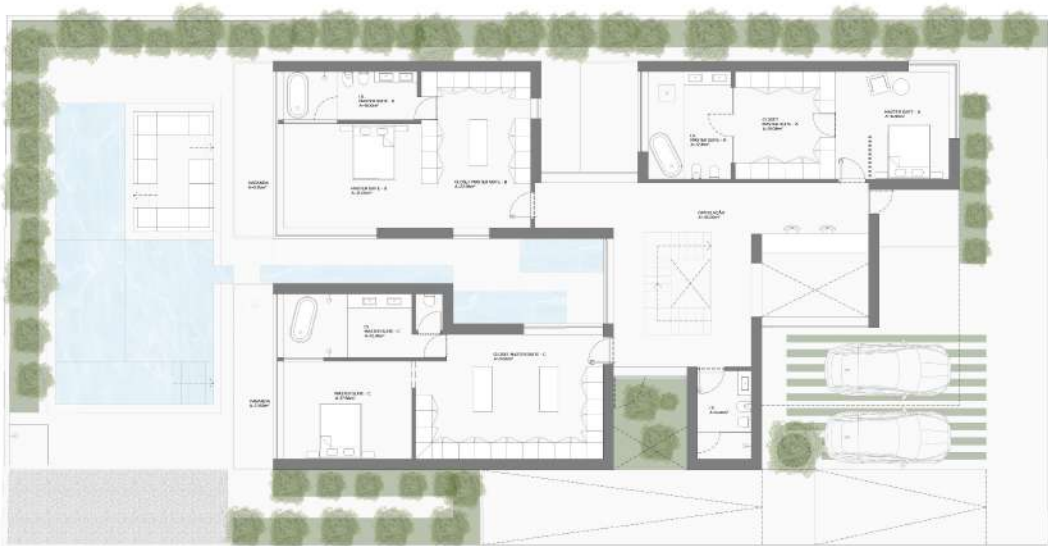
PLANTA PISO 1
