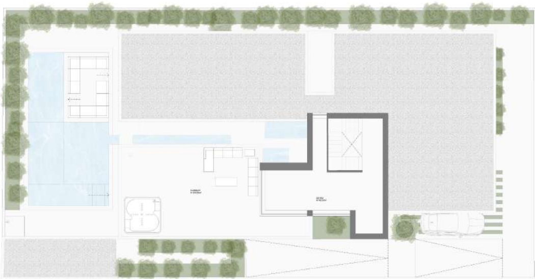
PLANTA PISO SÓTÃO / TERRAÇO
