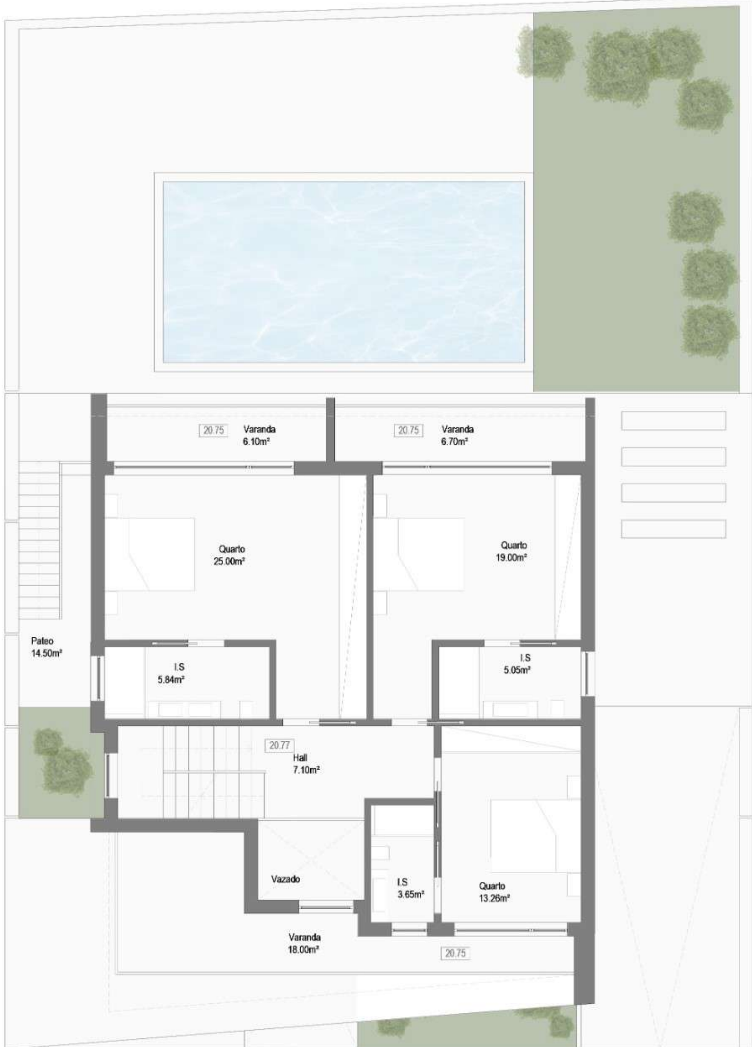
Planta do 1º Andar
