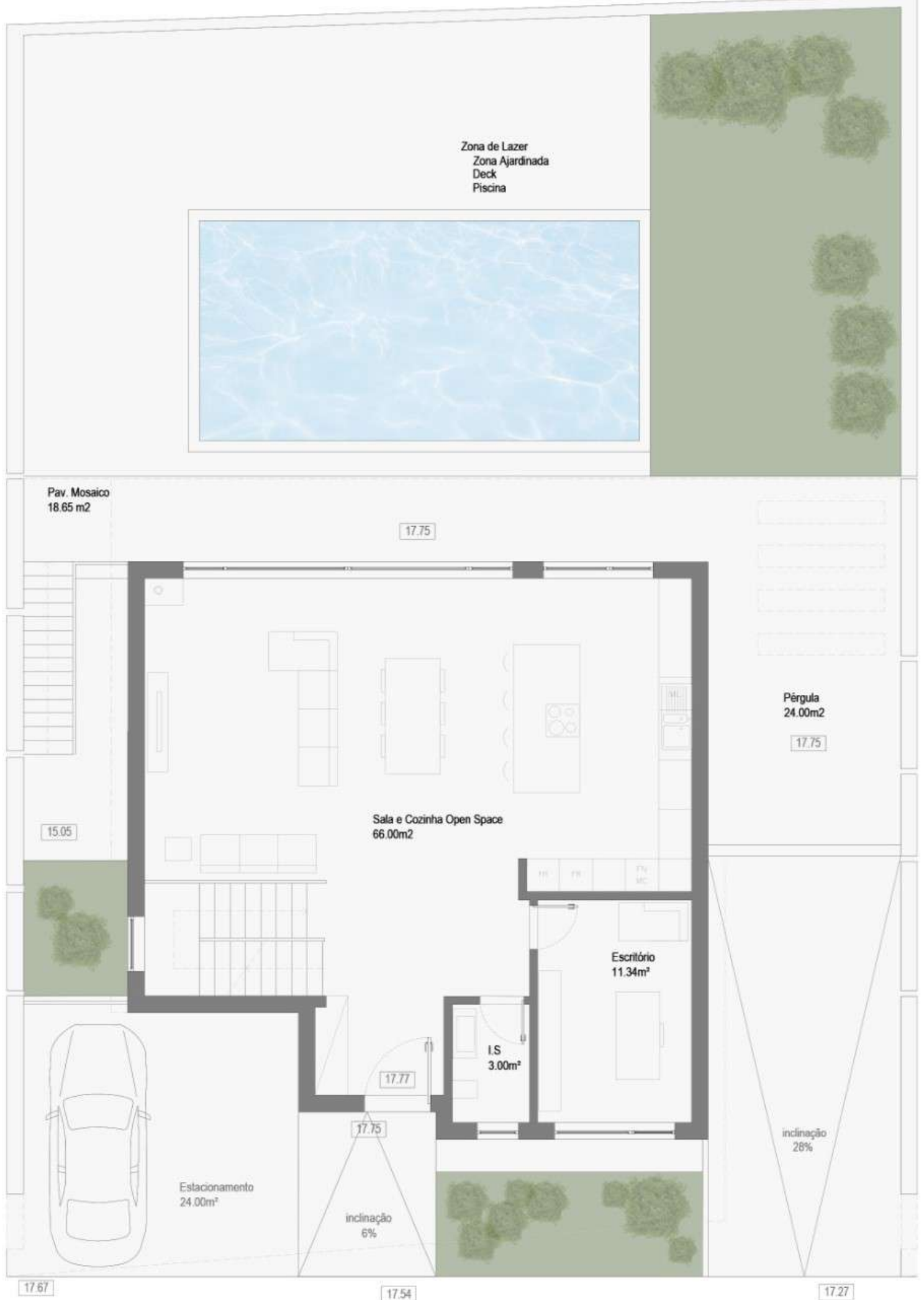
Planta do R/C
