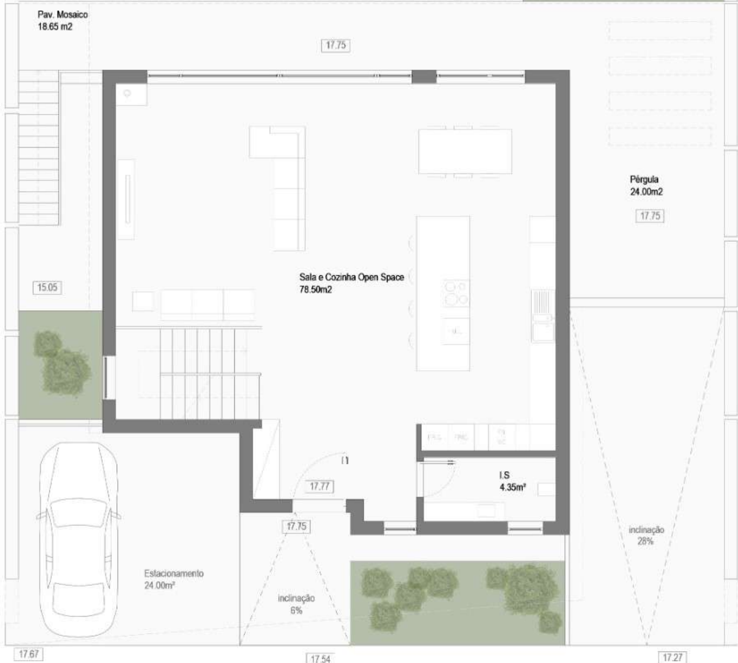
Planta do R/C
