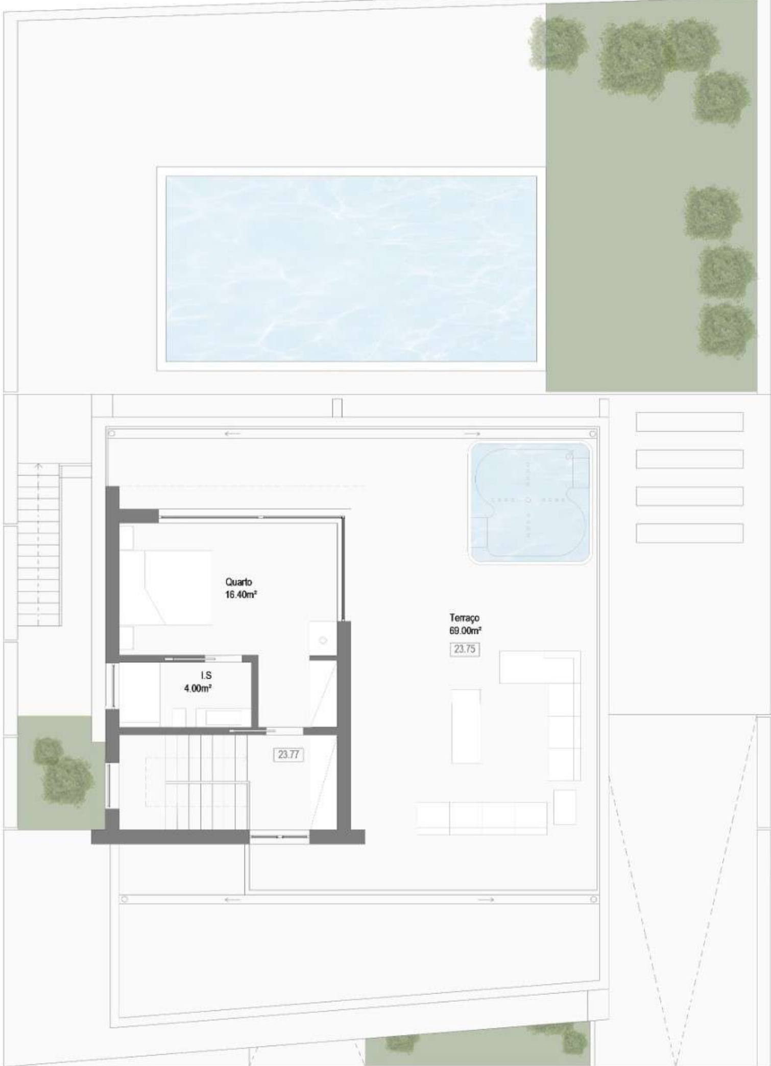
Planta do Sotão
